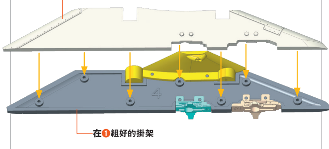
76-5 掛架零件5 (零件上有3的刻印)
